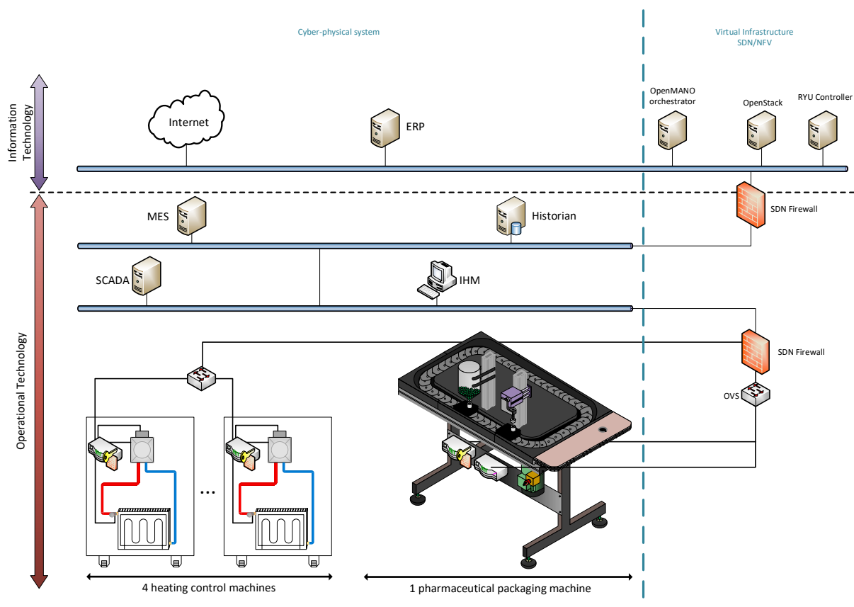
Figure 2. Plateforme Industrie 4.0 à l'université de Bretagne Occidentale
