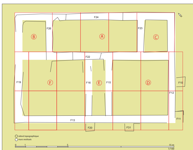
Fig. 27 : Proposition de restitution du tracé régulateur du bâtiment (Erwan Bourhis et Romuald Ferrette).
