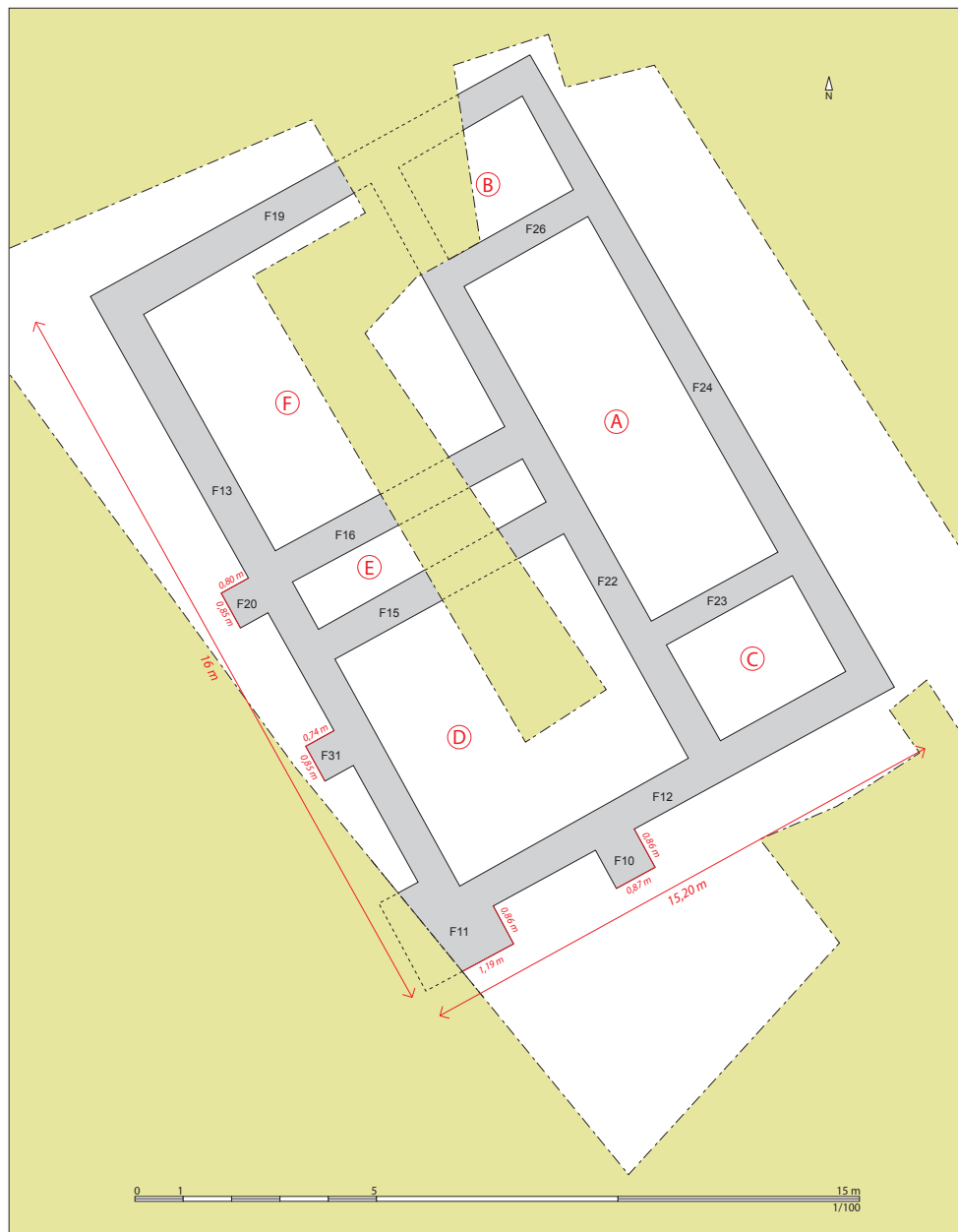
Fig. 7 : Plan général du bâtiment au 1/100 e (Erwan Bourhis).
