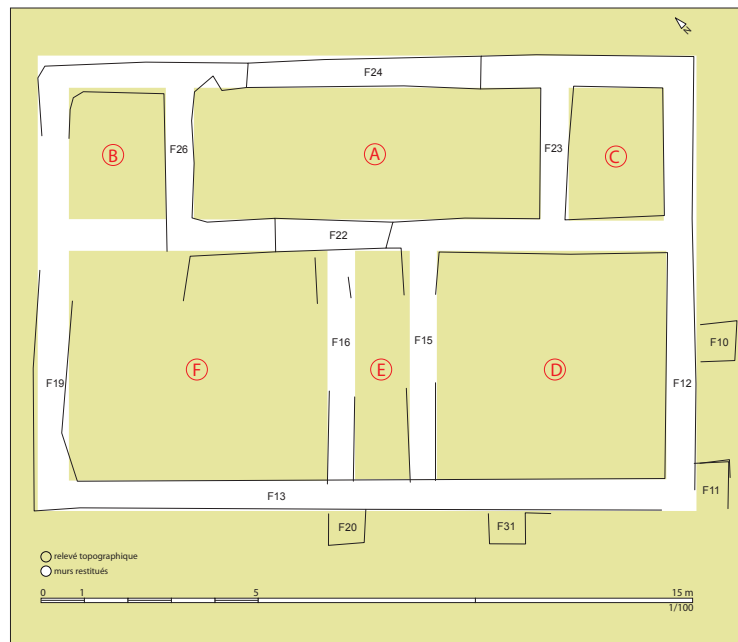
Fig. 23 : Restitution du plan de l'édifice à partir du levé topographique (Erwan Bourhis et Romuald Ferrette).
