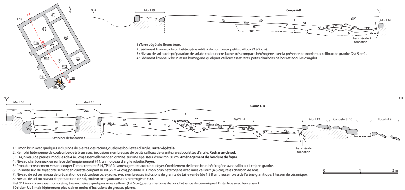
Fig. 21 : Coupe longitudinale du bâtiment (Erwan Bourhis).
