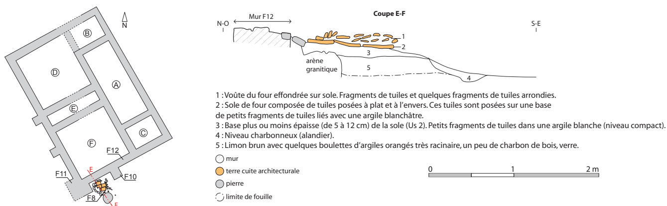
Fig. 19 : Localisation et coupe du four F8 (Erwan Bourhis).
