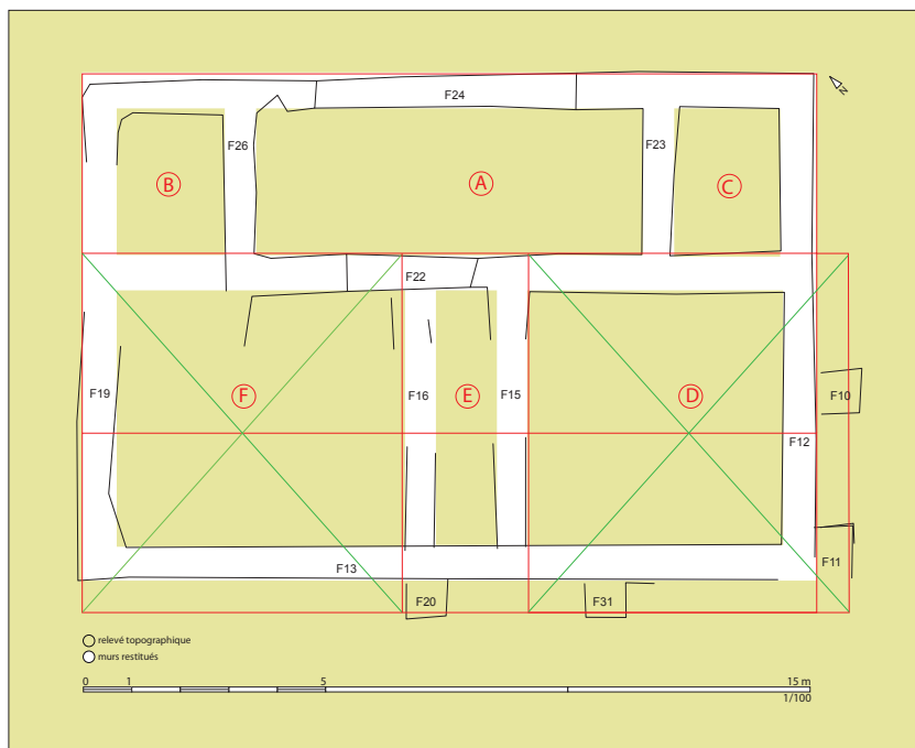
Fig. 25 : Mise en évidence de rapports proportionnels simples au sein de l'édifice (Erwan Bourhis et Romuald Ferrette).
