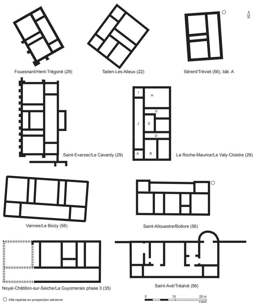
Fig. 28 : Planche comparative rassemblant des établissements qui entretiennent une parenté étroite avec le bâtiment de Hent Trégoné (Erwan Bourhis).
