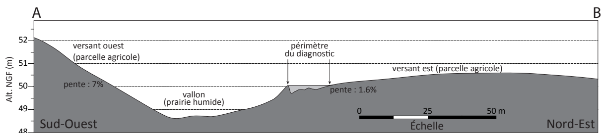
Fig. 4 : Profil topographique du secteur (Pierre Stéphan).
