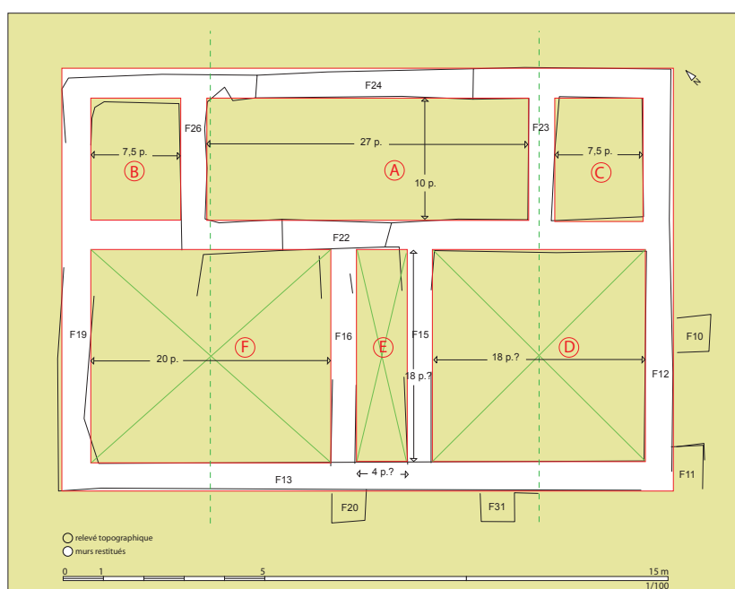
Fig. 26 : Les mesures intérieures des pièces exprimées en pieds (Erwan Bourhis et Romuald Ferrette).
