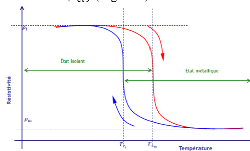
Figure 1. Hystérésis d'évolution des propriétés électriques du VO 2 pour une commande thermique [6]
