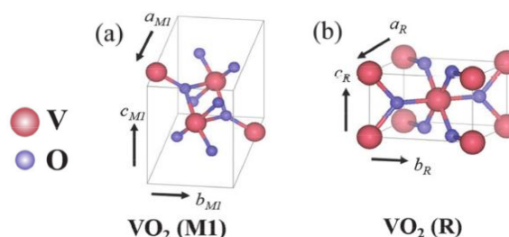
Figure 2. Structures cristallines polymorphes du VO 2 : a) monoclinique isolante M1 et b) rutile métallique R [7]
