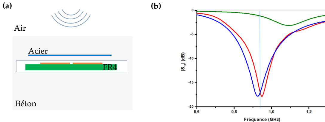
FIGURE 1. (a) schéma du capteur RFID. (b) simulations électromagnétiques du paramètre de réflexion S_{11} de l'antenne dipolaire dans des bétons secs et saturés en eau de mer (courbe rouge et bleue), soumise à l'interaction d'une couche métallique dans le béton sec (courbe verte).
