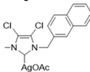
Ag-NHC 12
