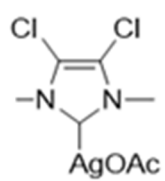
Ag-NHC 5
