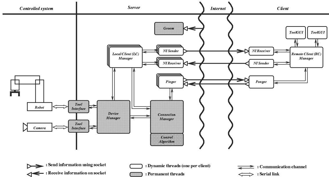
FIG. 3 – architecture logicielle générique
