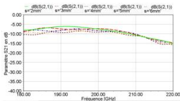
Figure 9 : paramètres de transmission S21 simulés entre deux dipôles sur un substrat silicium et pour différentes distances entre les antennes.
