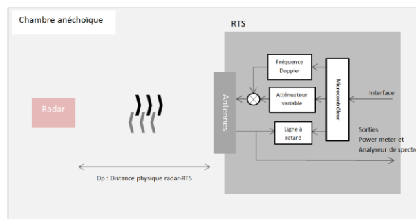
Figure 1. Synoptique d'un simulateur de cibles radar (RTS)
