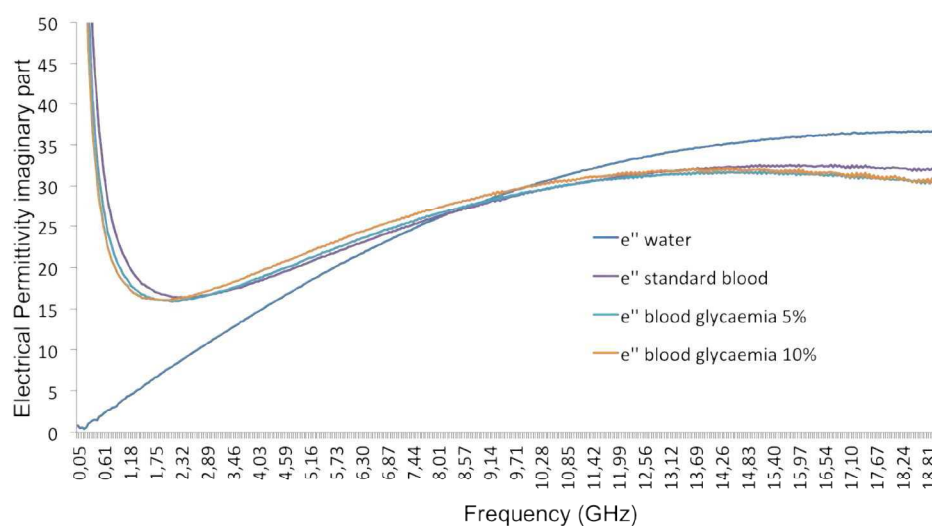
Figure 2. Permittivités diélectriques relatives relevées pour du sang humain avec différentes glycémies (a/ partie réelle, b/ partie imaginaire).
