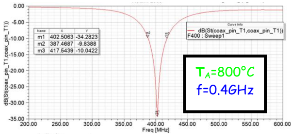
Figure 3b. Coefficients de réflexions (HFSS) d'antennes patch réalisées sur le matériau S2 ( T_A=800^\circ\text{C} ).
