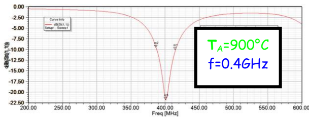
Figure 3a. Coefficients de réflexions (HFSS) d'antennes patch réalisées sur le matériau S3 ( T_A=900^\circ\text{C} ).
