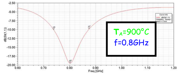
Figure 3a. Coefficients de réflexions (HFSS) d'antennes patch réalisées sur le matériau S3 ( T_A=900^\circ\text{C} ).
