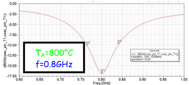
Figure 3b. Coefficients de réflexions (HFSS) d'antennes patch réalisées sur le matériau S2 ( T_A=800^\circ\text{C} ).
