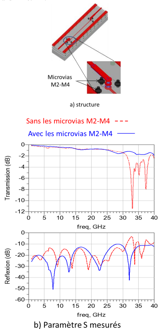
Figure 4: a) position des plots reliant les plans de masse M2 et M4 ; b) paramètres S mesurés avec et sans la présence de ces plots.
