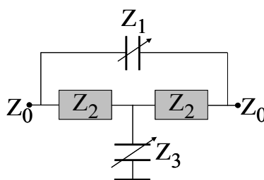
Figure 2 : déphaseur passe-tout
