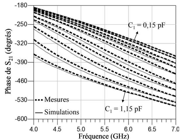
Figure 4. Comparaison des phases mesurées et simulées.
