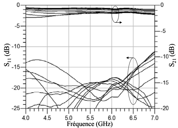
Figure 3. Paramètres S mesurés.
