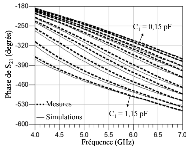
Figure 4. Comparaison des phases mesurées et simulées.
