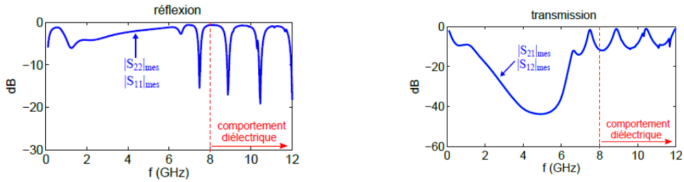
Figure 5 : Paramètres S mesurés d'un ferrite spinel désaimanté : comportement diélectrique haute fréquence
