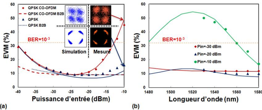
Figure 3 : (a) EVM simulée (ligne continue) et mesurée (points) et constellations du signal reçu en fonction de la puissance d'entrée SOA pour des signaux QPSK et QPSK CO-OFDM à la longueur d'onde de 1540 nm (b) EVM d'un signal QPSK CO-OFDM simulé (ligne continue) et mesuré (points) en fonction de la longueur d'onde pour trois puissances injectées dans le SOA (-30, -20, -10 dBm). Le courant de polarisation est de 200 mA. B2B: Back-to-Back (même chaîne de transmission mais sans le SOA).
