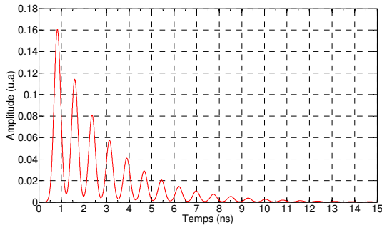
Figure 3. Impulsion optique modulée à 1,3 GHz
