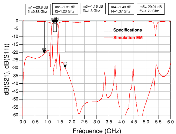
Figure 8. Simulation EM du filtre
