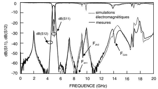
Figure 9 Simulations électromagnétiques et mesures du second filtre modifié d'ordre 4.
